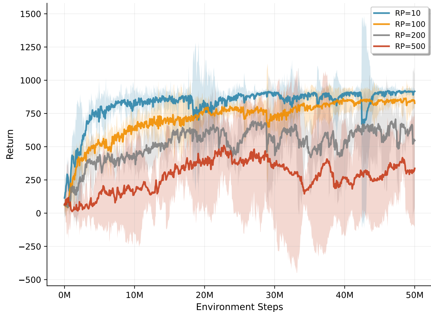
IPPO
