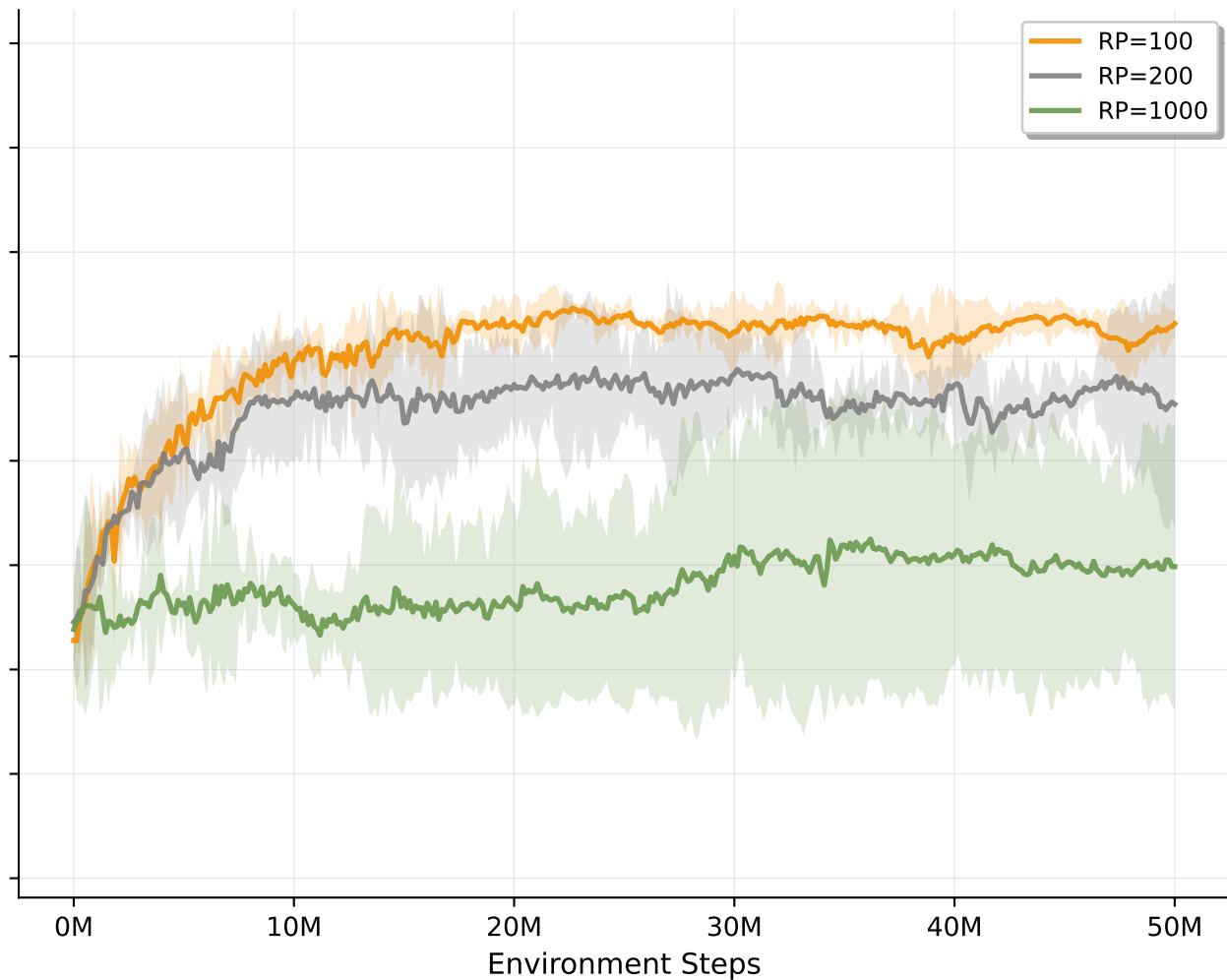
MAPPO
